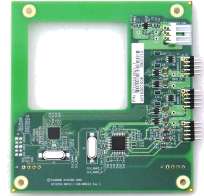
Концентратор аудио и USB Дисплей пассажира автобуса
