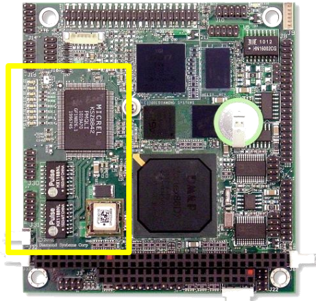
Заказной ввод-вывод #1 Коммутатор Ethernet
