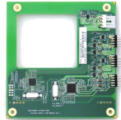
Аудиоплата по индивидуальному заказу
